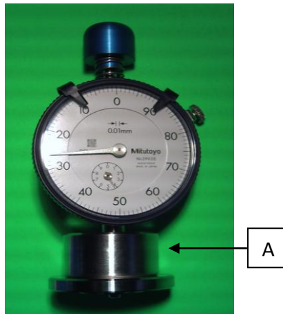
图 2: 校正方法
